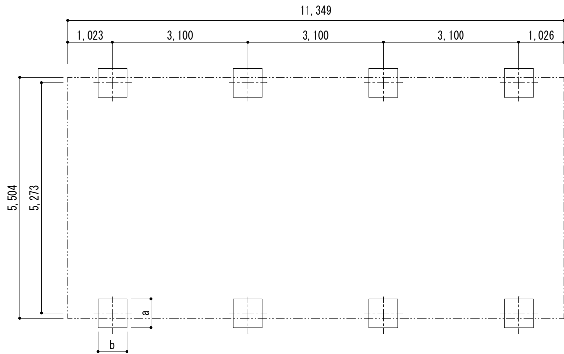
■基礎配置図
